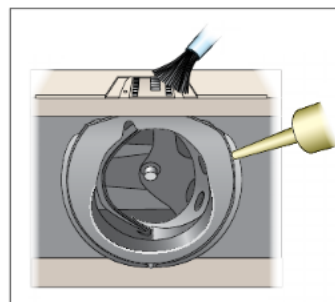
Рис. 48. Чистка и смазка швейной машины
