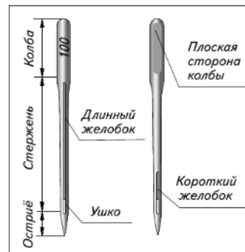
Рис. 43. Машинная игла
